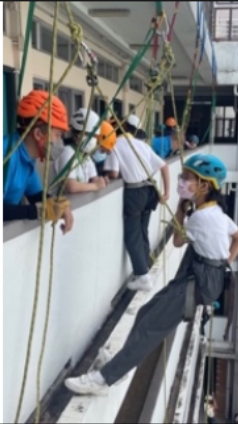
親子同步緣繩下降
